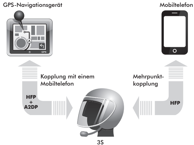
Kopplung des GPS-Navigationsgeräts als Mobiltelefon
