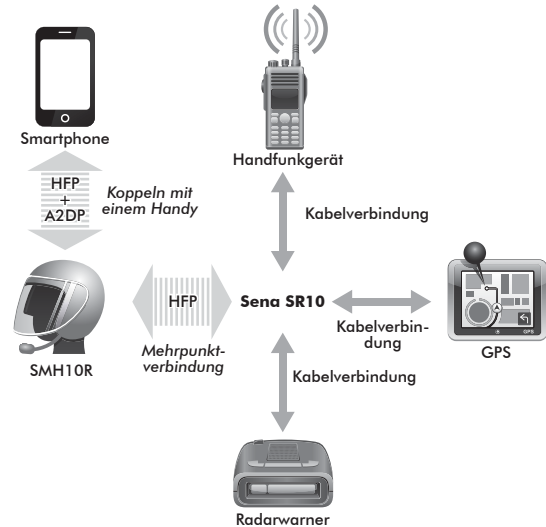
Parallele Verbindung des SR10 und des Handys per Bluetooth-Mehrpunktkopplung
